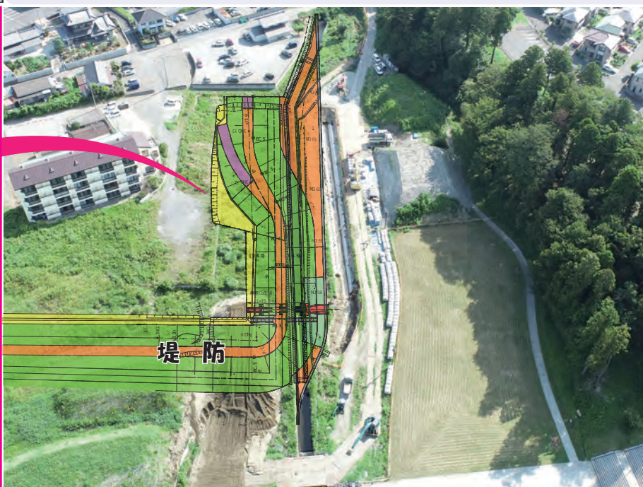
▲工事前の一級河川中丸川▶下流部の洪水吐施設の整備状況
